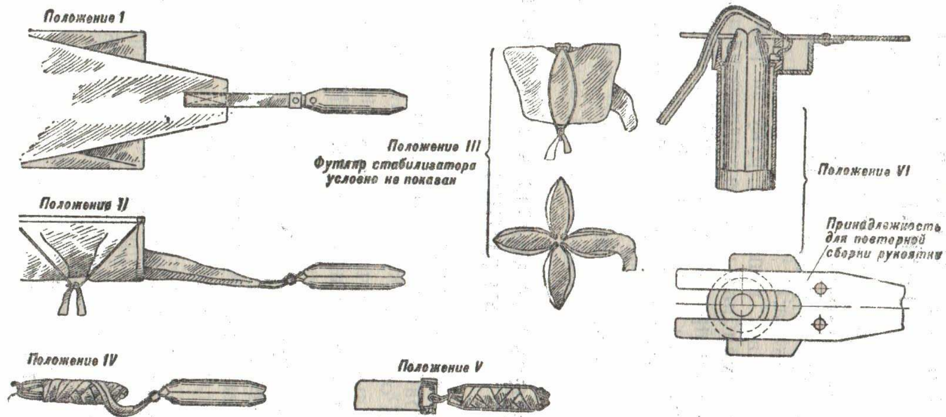
Рис. 4. Схема укладки стабилизатора
