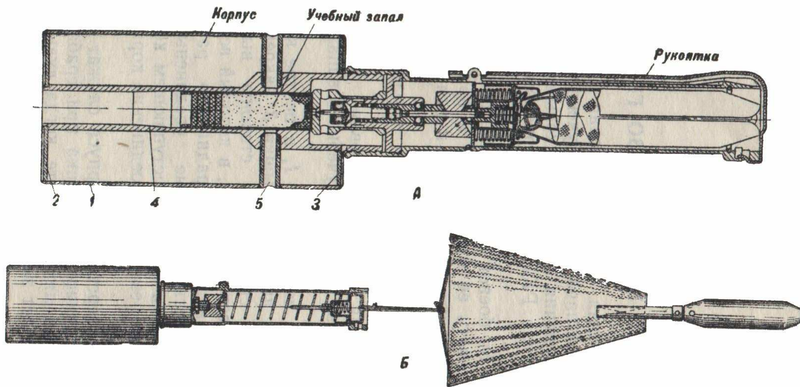
Рис. 1. Учебная ручная противотанковая граната: А — устройство гранаты: 1 — оболочка; 2 — дно; 3 — крышка; 4 — ствол; 5 — трубка; Б — граната в полете
